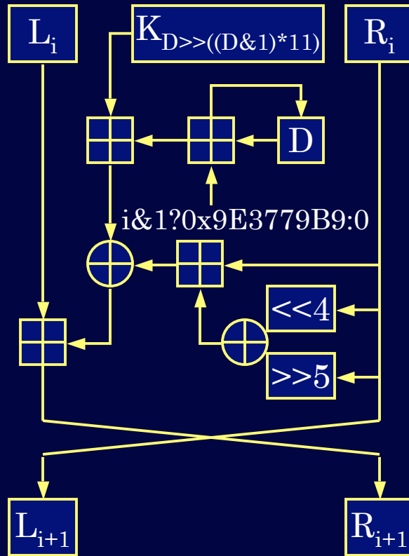
XTEA: 9/19
